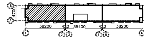
Блокировочная схема
