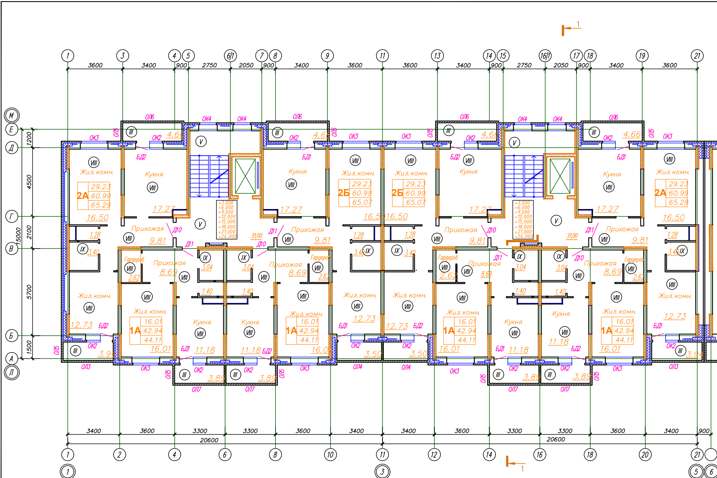
Экспликация помещений квартир типа 2.А
